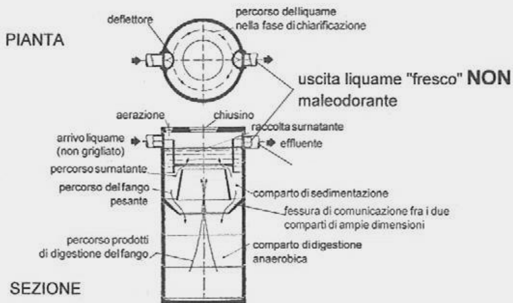
Fig. 5 - Tipo di fossa Imhoff adatta per utenze individuali (fossa settica-Imhoff)
