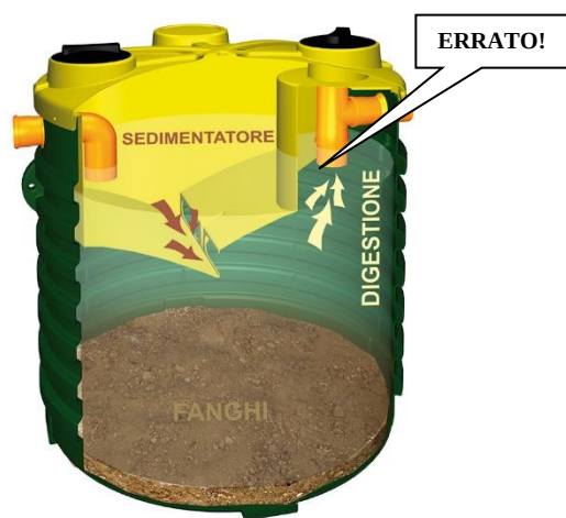
SCHEMA TECNICO 4
