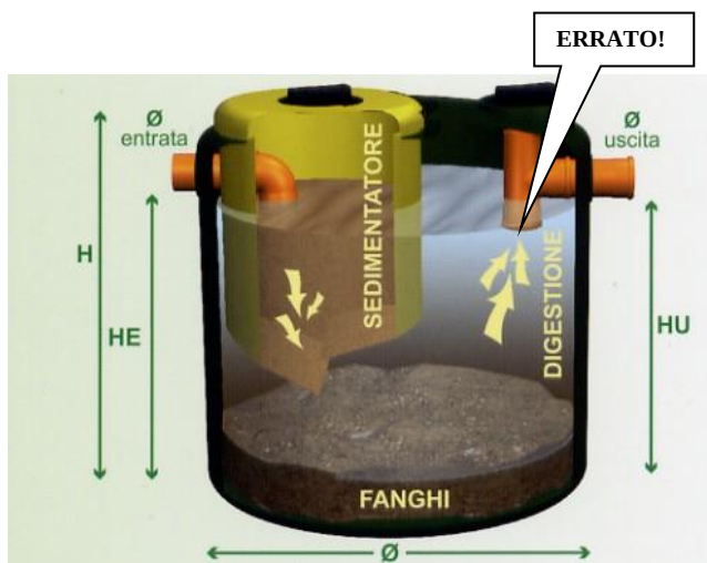
SCHEMA TECNICO 3
