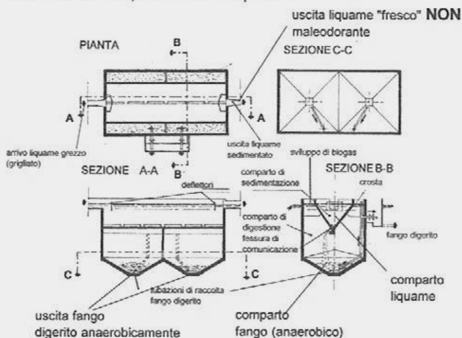
Fig. 3 - Pianta e sezione di fossa Imhoff
