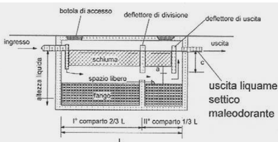
Fig. 2 Fossa settica bicamerale
