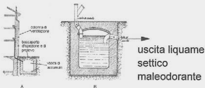
Fig. 1-A) Pozzo nero posto alla base degli scarichi di un'abitazione; B) Modifica introdotta dal francese Jean Louis Mourras de Vesoul con trasformazione del pozzo nero in fossa settica.
